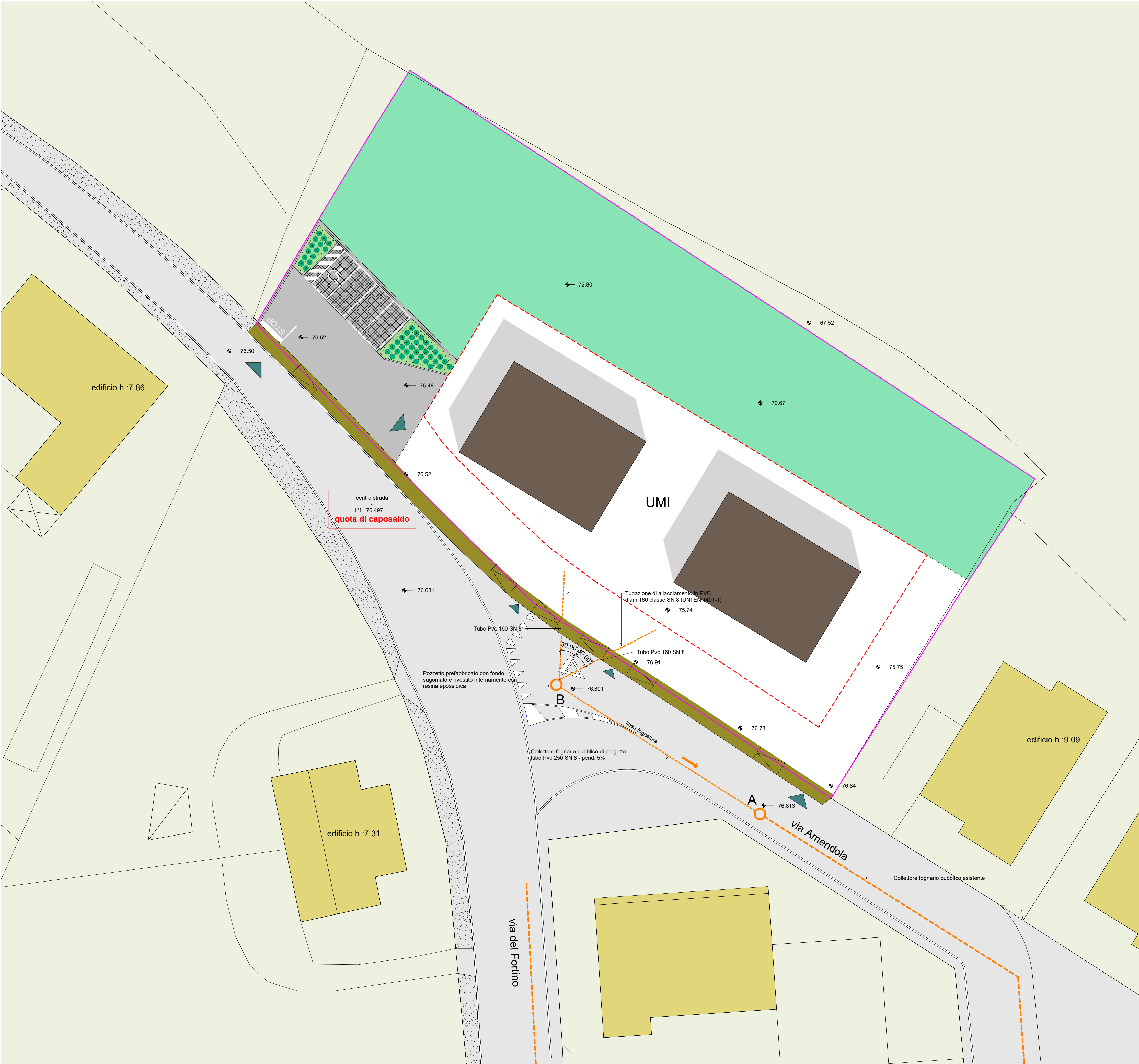
Planimetria scala 1:200
